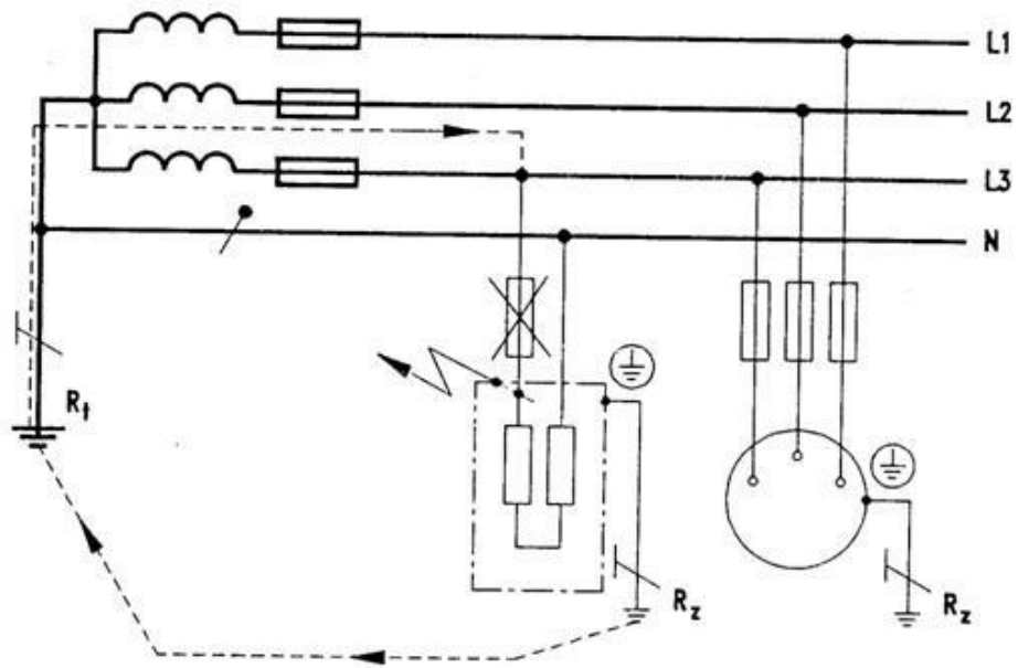
Obr. 13.8 Princip ochrany samočinným odpojením od zdroje v síti TT
